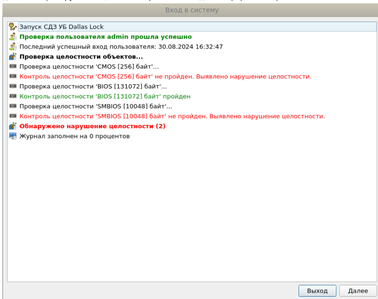
Рис. 24. Пример окна сообщения при неуспешном прохождении контроля целостности при входе пользователя
