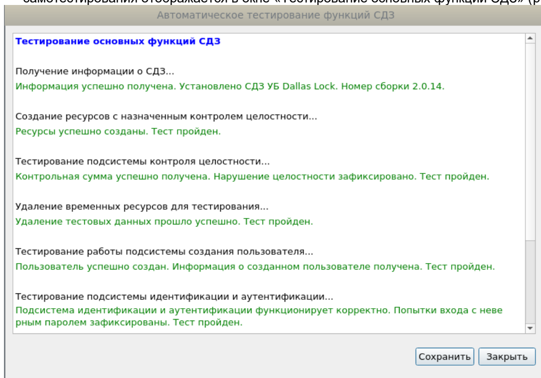
Рис. 78. Окно результатов тестирования основных функций СДЗ
