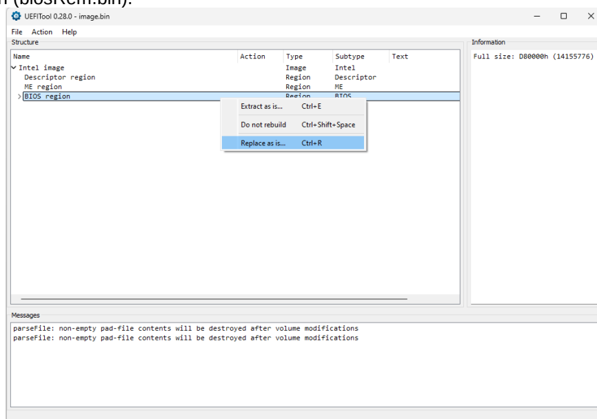
Рис. 7. Дерево элементов BIOS. Замена элемента «BIOS region»
