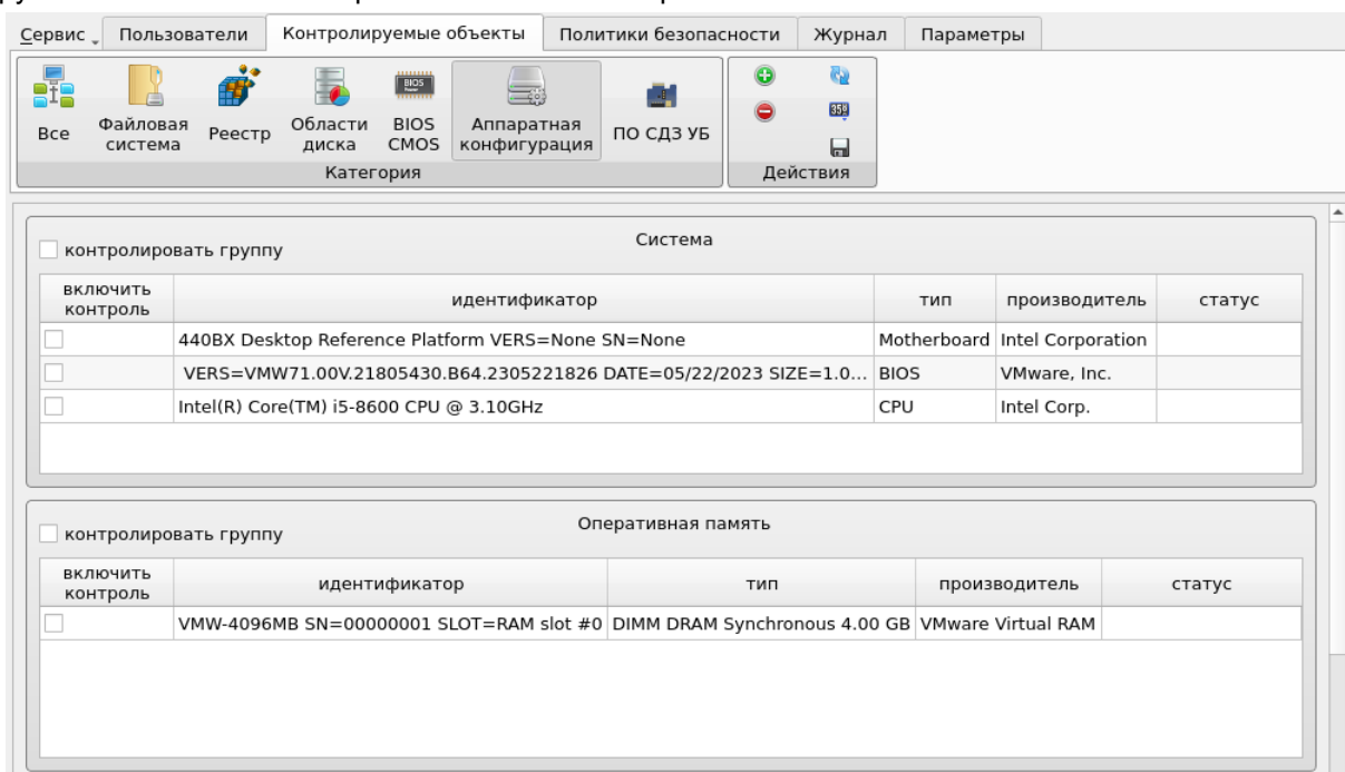
Рис. 62. Главное окно. Контролируемые объекты аппаратной конфигурации ТС
