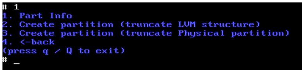
Рис. 3. Опции ручного режима создания раздела программы PartitionTool
